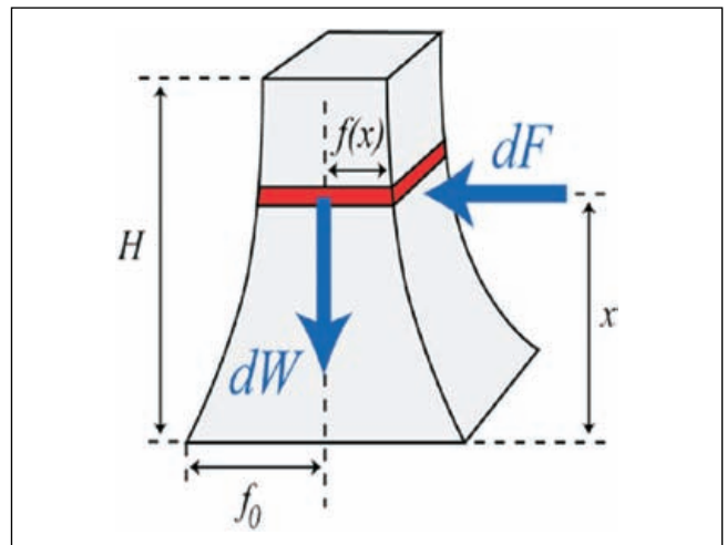
Figura 40. Perfil f(x) de las aristas, resultantes elementales del peso y del viento vertical.
