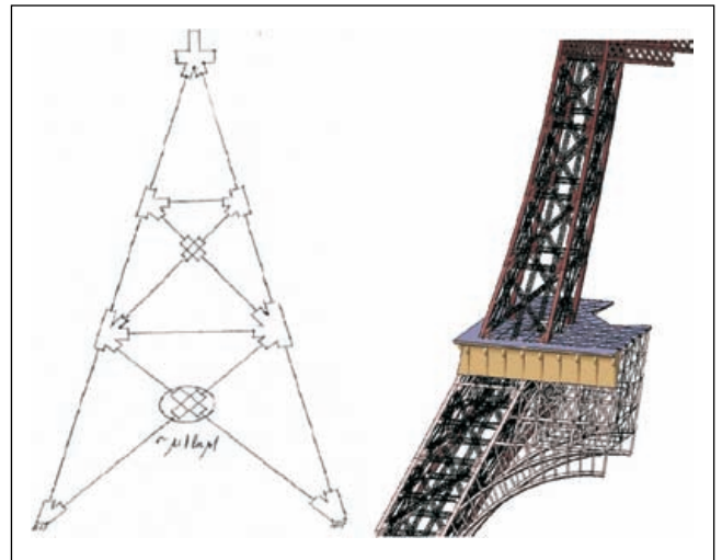
Figura 44. Torre híbrida con elementos de diferentes dimensiones espaciales (tomado del texto de Panasenko) y representación de la estructura híbrida con el programa CATIA.
