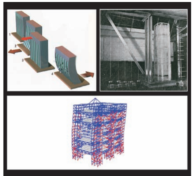
Figura 27. Movimientos sísmicos y su estudio en modelos analógicos e informáticos.
