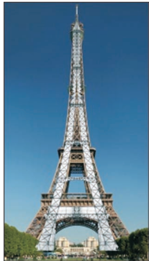
Figura 39. Superposición del diseño primitivo y la torre actual 40 .
