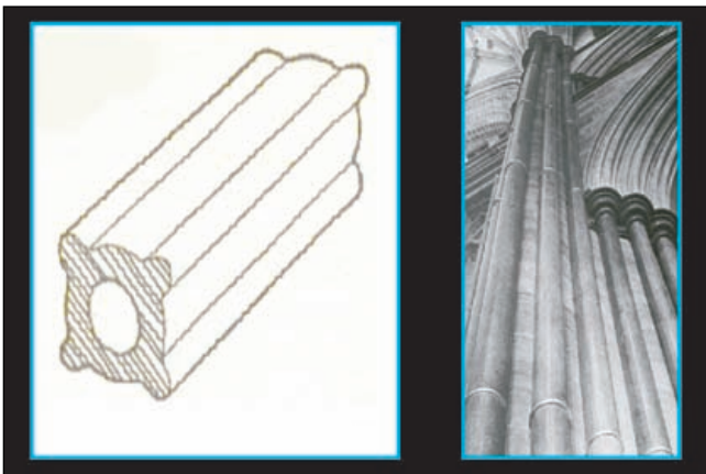
Figura 33. Columnas reforzadas por yuxtaposición de elementos básicos. Catedral de Salisbury.
